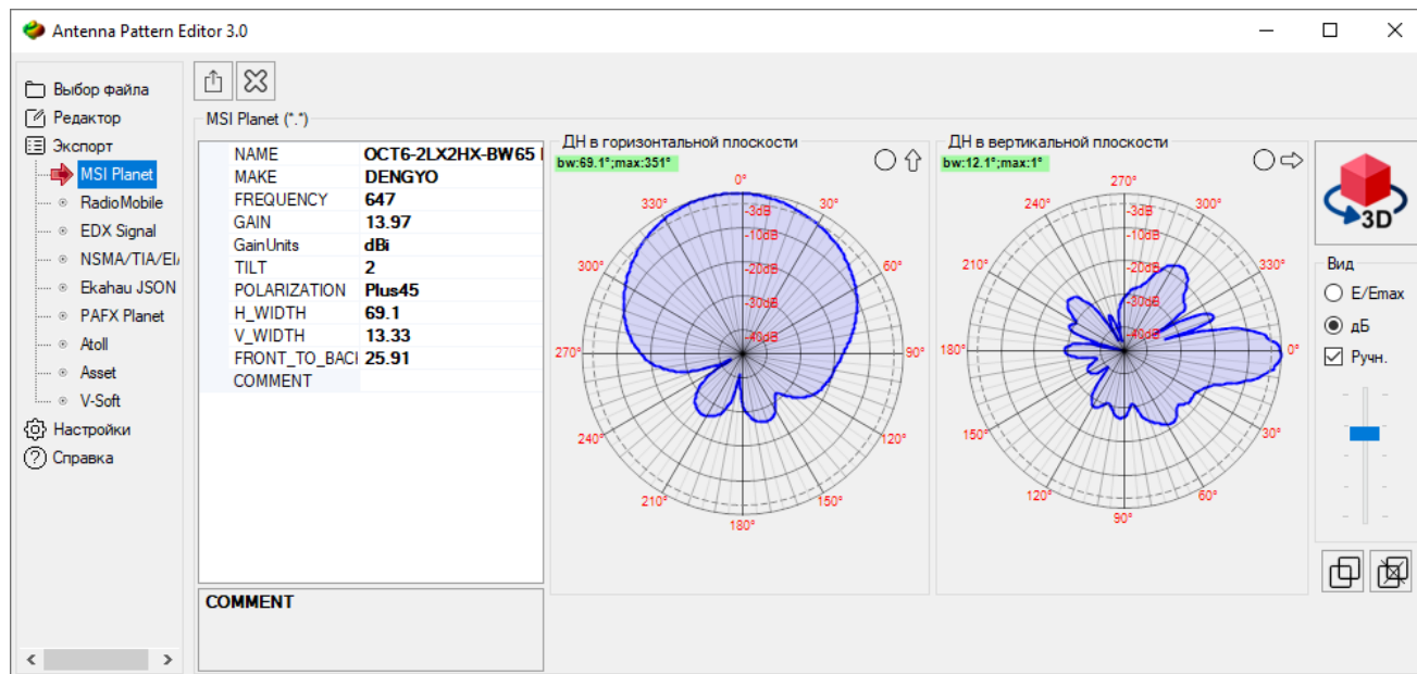
Экспорт диаграммы направленности антенны в файл MSI
